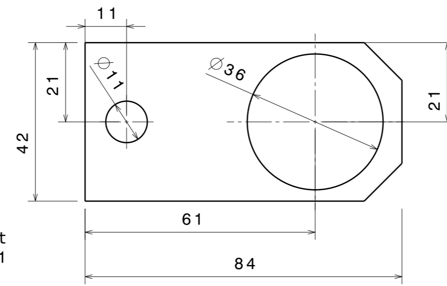
Seitenansicht links Maßstab: 1:1
