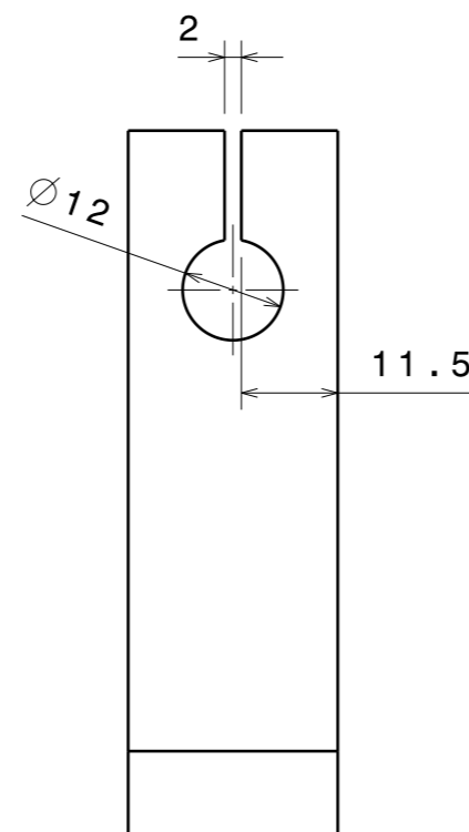
Draufsicht Maßstab: 1:1
