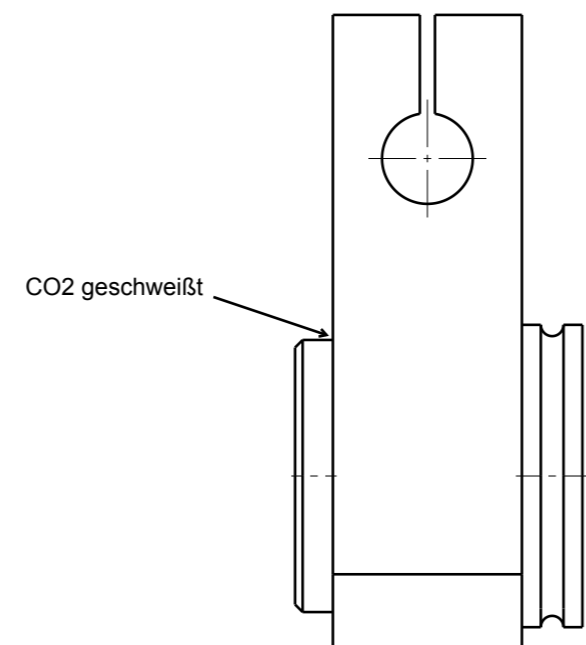
Draufsicht Maßstab: 1:1
