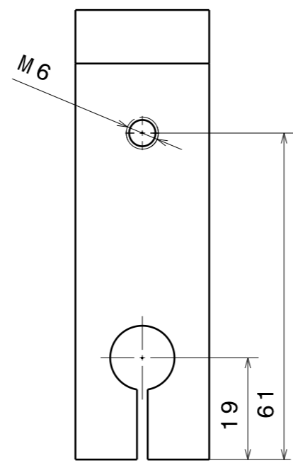
Untersicht Maßstab: 1:1
