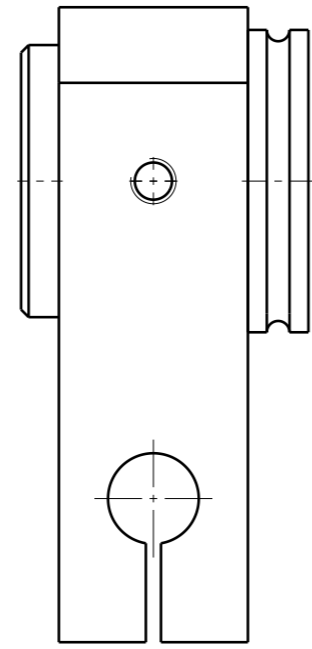
Untersicht Maßstab: 1:1
